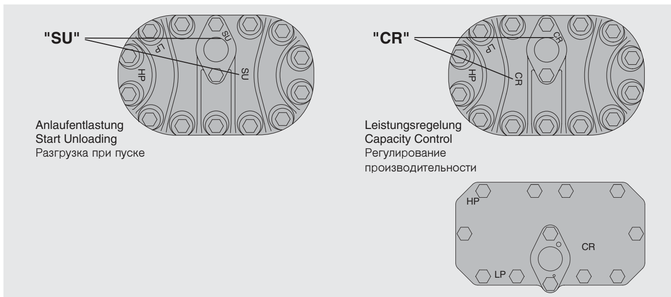
Abb. 4 Anlaufentlastung / Leistungsregelung
